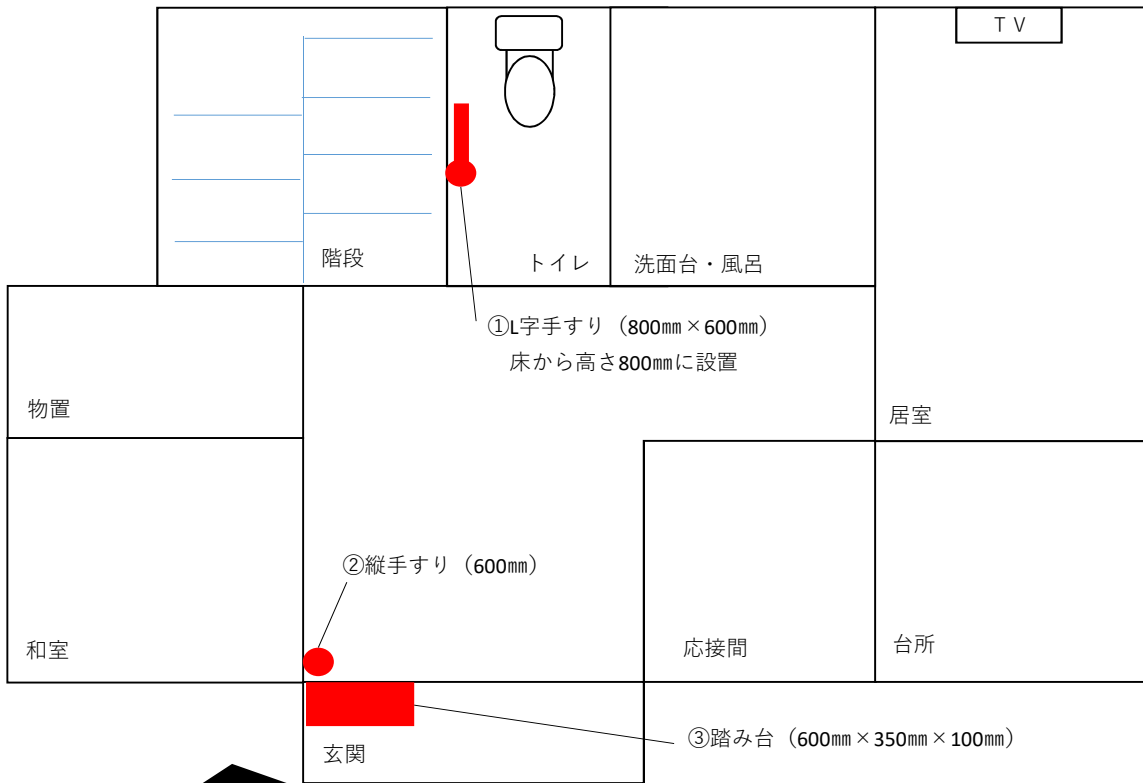
平面図 (例)
